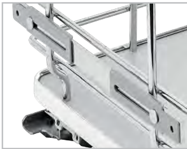
Features Rev-A-Shelf's patented AMB door mount brackets US Patent No. 7,204,569
