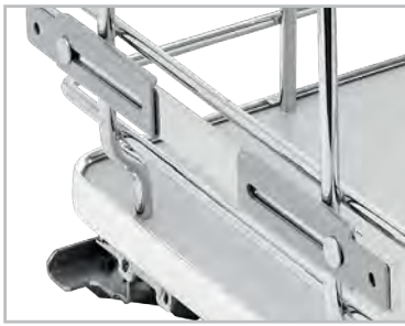
Features Rev-A-Shelf's patented AMB door mount brackets US Patent No. 7,204,569
